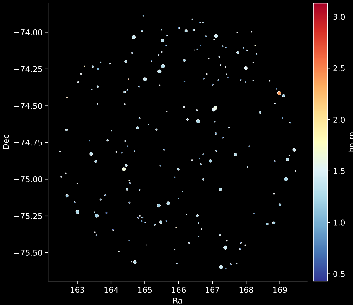
APOGEE DR17 Field: [288-35-O_TESS] Stars: 188
